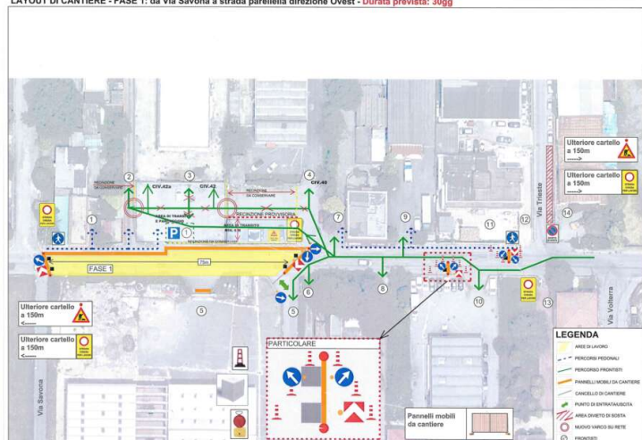
LAYOUT DI CANTIERE - FASE 1: da Via Savona a strada parallela direzione Ovest - Durata prevista: 30gg
